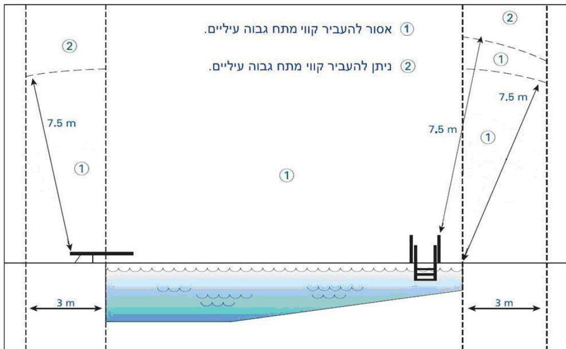
איור מס' 1: העברת קווי רשת עילית בקרבת בריכות שחייה
